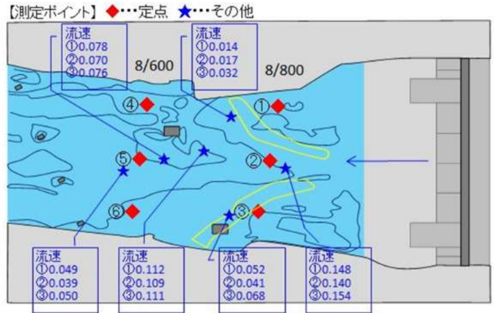
流速計測結果（平水流量）
